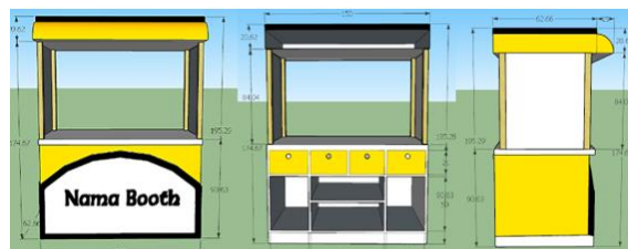
Gambar 6 Perencanaan booth
