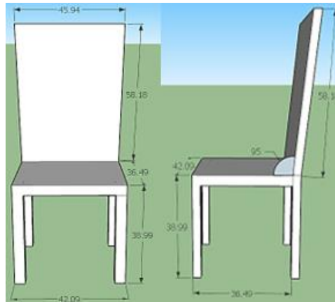
Gambar 4 Perancangan kursi makan
